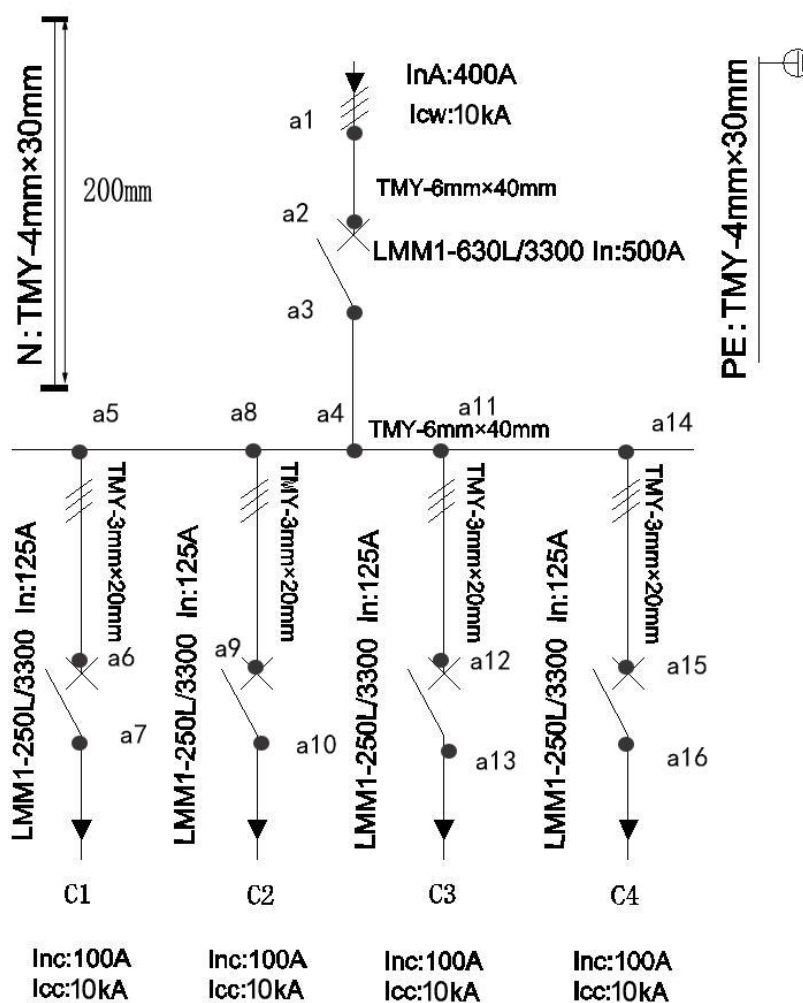
温升 (绝缘支撑件) 示意图编号: WS2300542001
